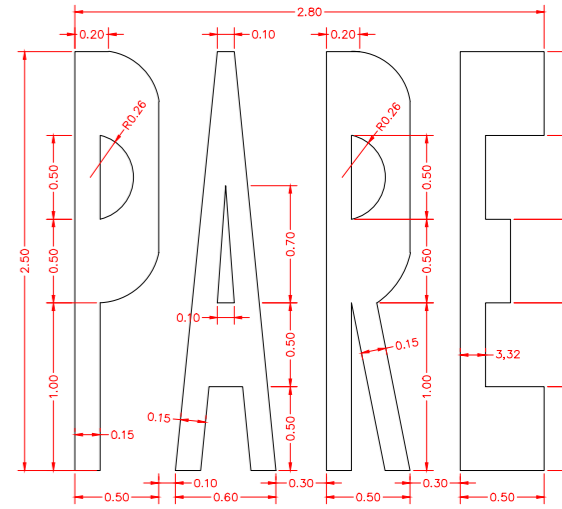
DEMARCACIÓN HORIZONTAL Tipo 10 Total Lámina: 20m
