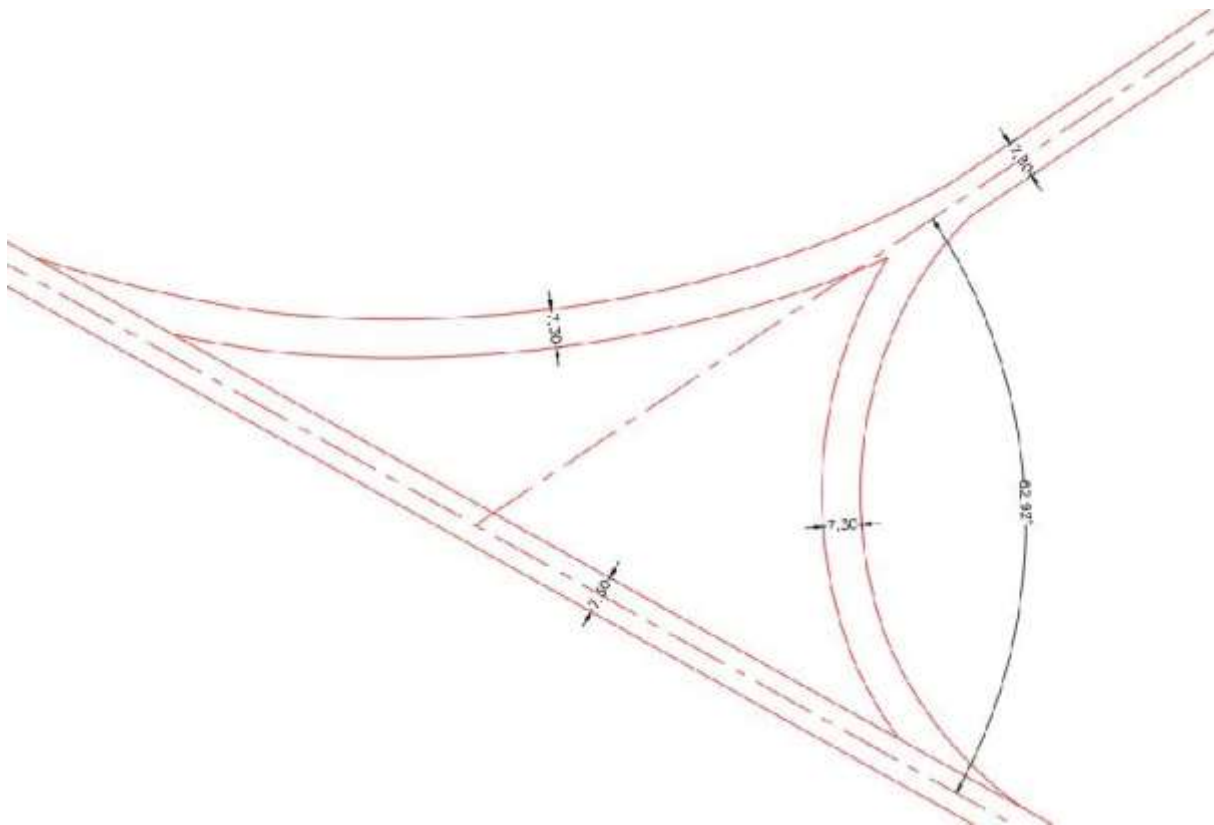
Imagen 5: Geometría Actual de Intersección
