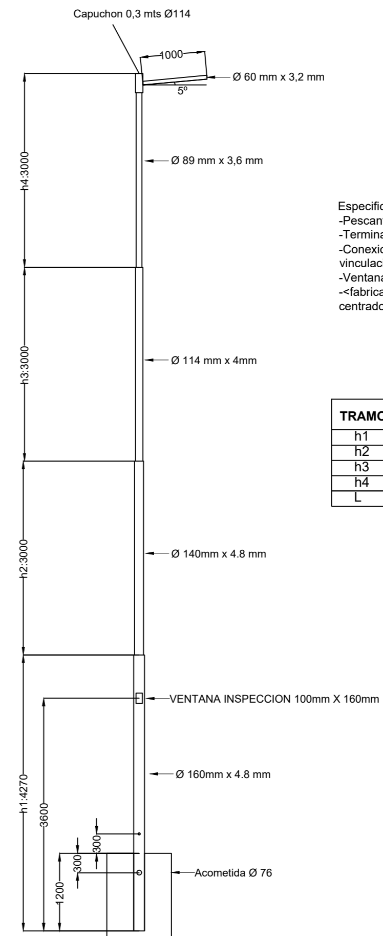
COLUMNA 12m CAPUCHON PESCANTE 1mts
